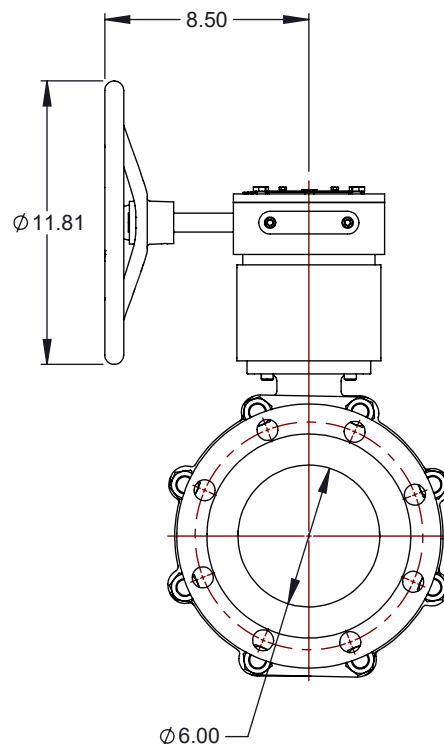
ISO 5211-F12
